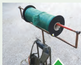
Cacolet pour la mise en place des filets de protection
